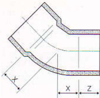
45° ELBOW B
